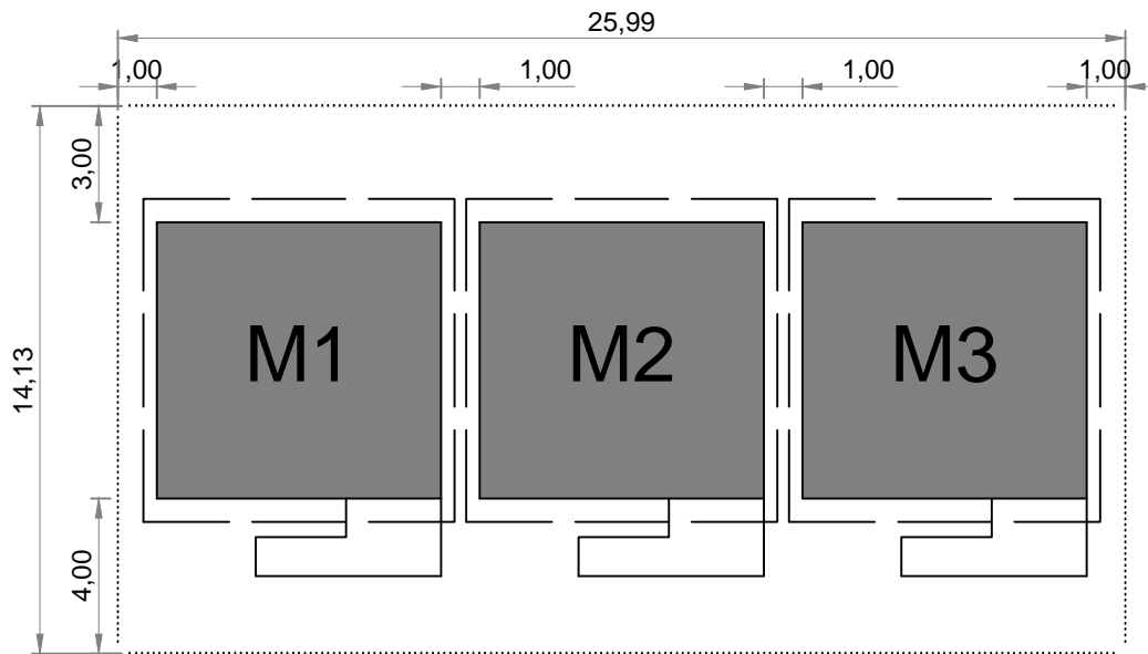
ESPACIO MINIMO PARA LA INSTALACION 3 MODULOS
