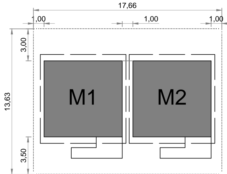
ESPACIO MINIMO PARA LA INSTALACION 2 MODULOS
