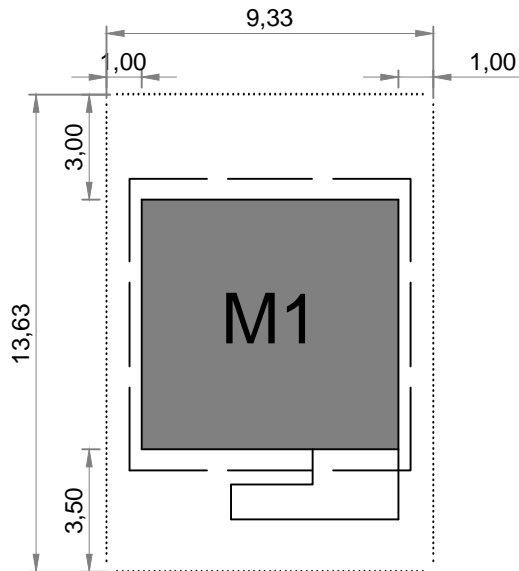
ESPACIO MINIMO PARA LA INSTALACION 1 MODULO
