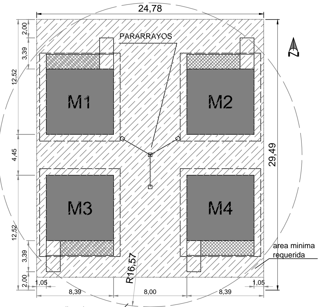
4 MODULOS
