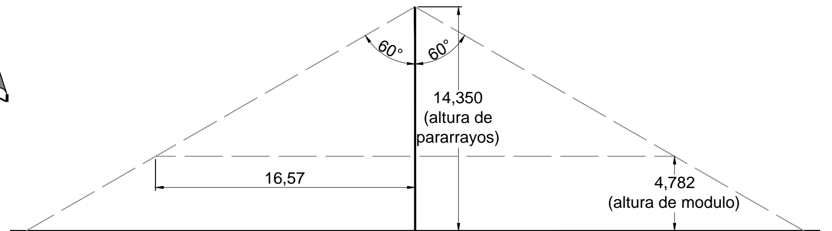
ESQUEMA COBERTURA DE PARARRAYOS
