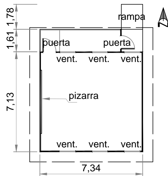
AULA PREFABRICADA
