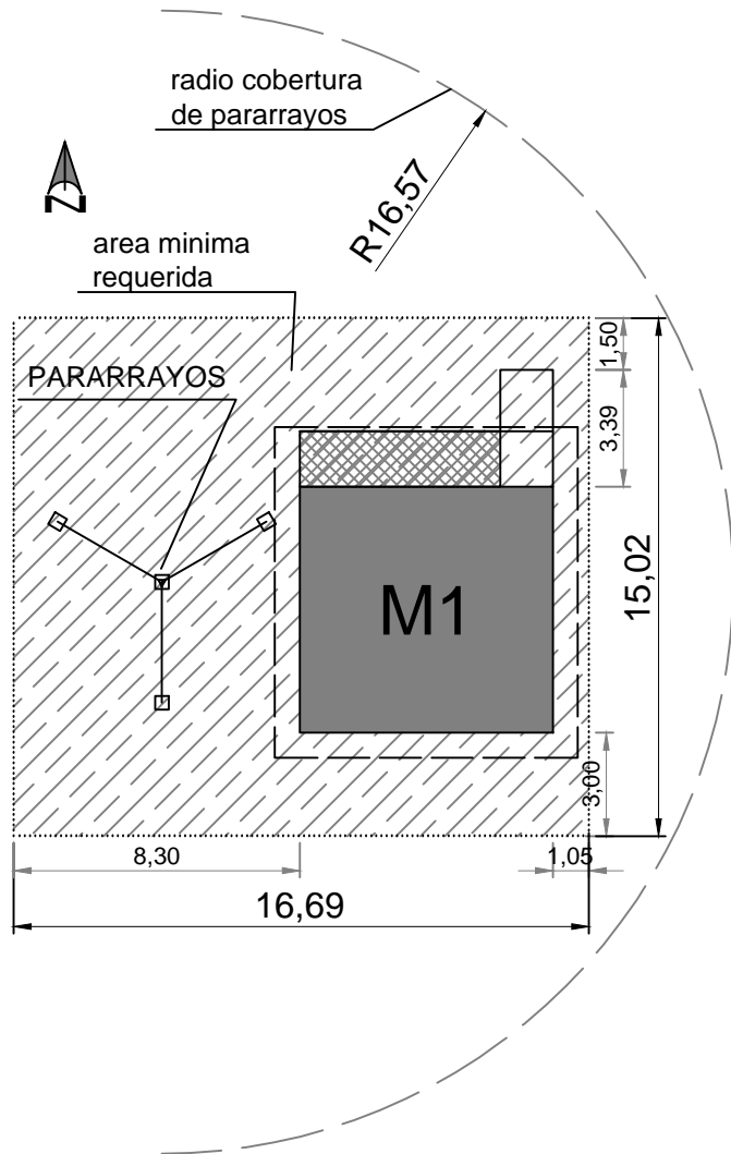
1 MODULO
